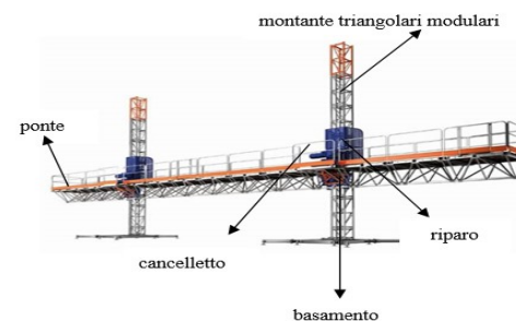
Piattaforma da lavoro elevabile su colonne PLAC
