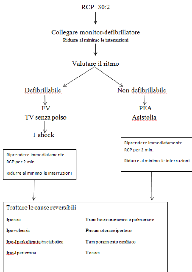
Fig. 1. ALGORITMO RCP 2015.
