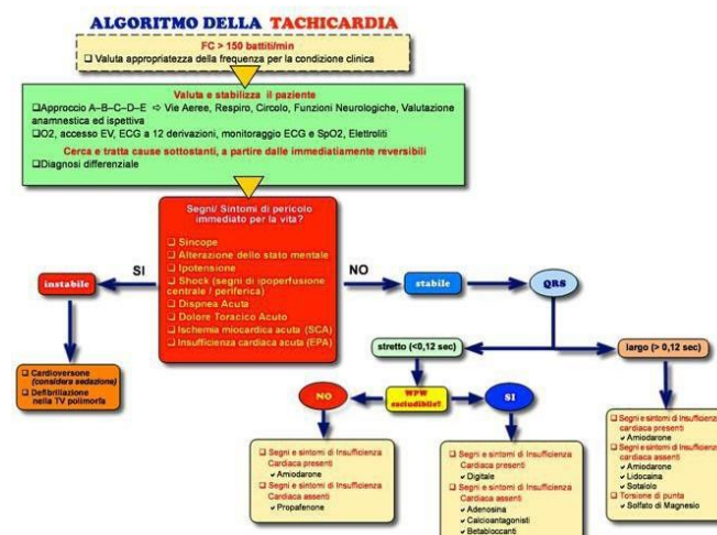
Fig. 1. TACHICARDIA: Algoritmo 2015
