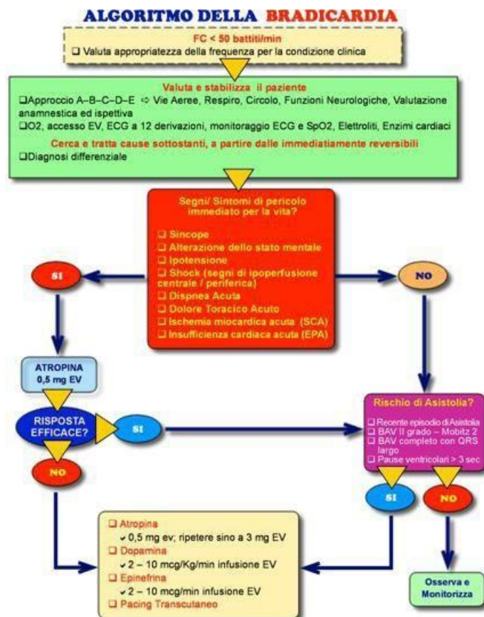
Fig. 2: BRADICARDIA: Algoritmo 2015
